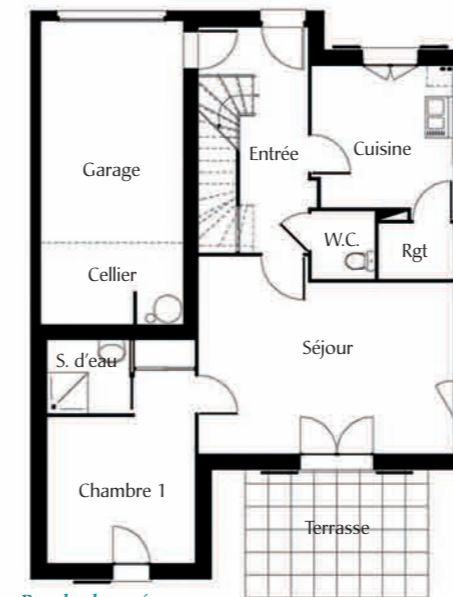
Rez-de-chaussée
