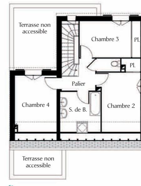
Etage
