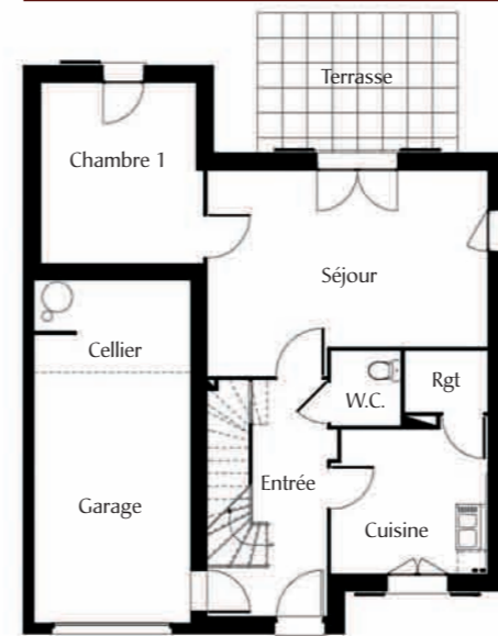
Rez-de-chaussée
